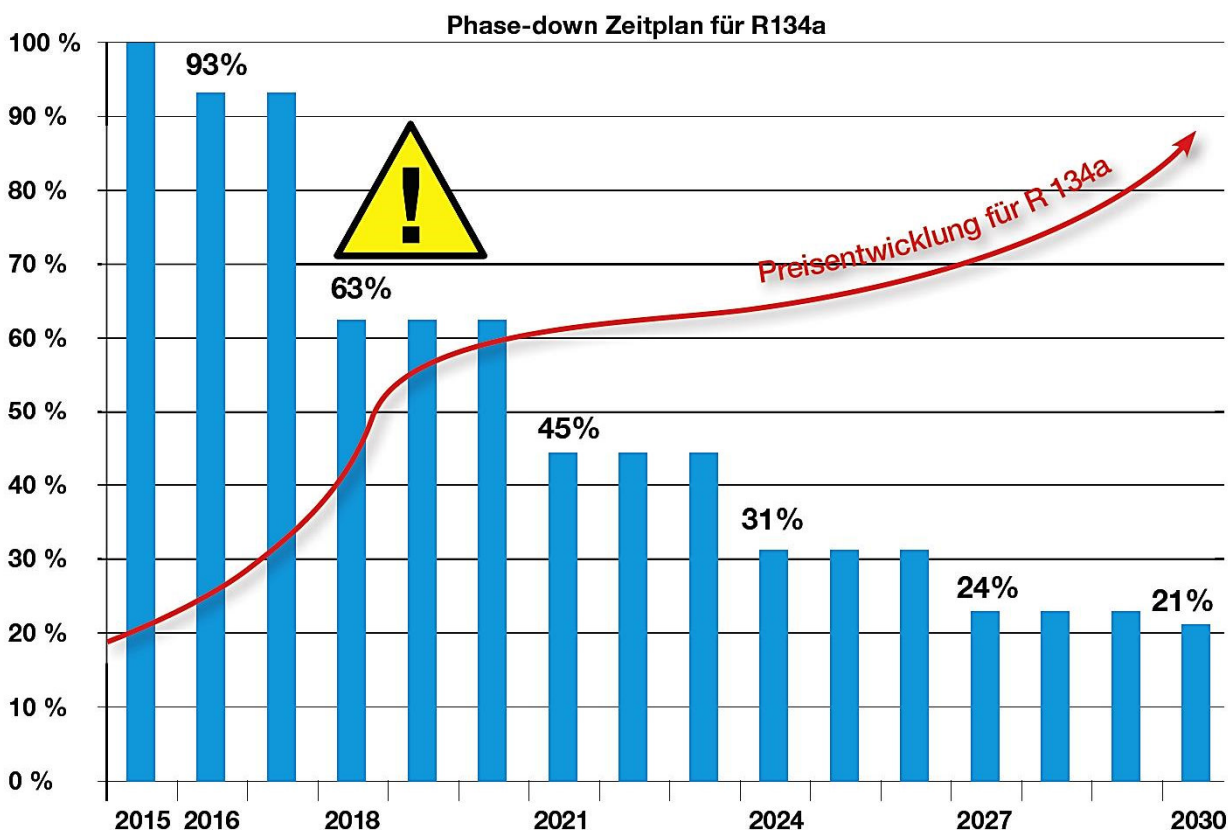
Abbildung: Phase-Down Zeitplan und prognostizierte Preisentwicklung für das Kältemittel R134a (Quelle: European Partnership for Energy and the Environment)
